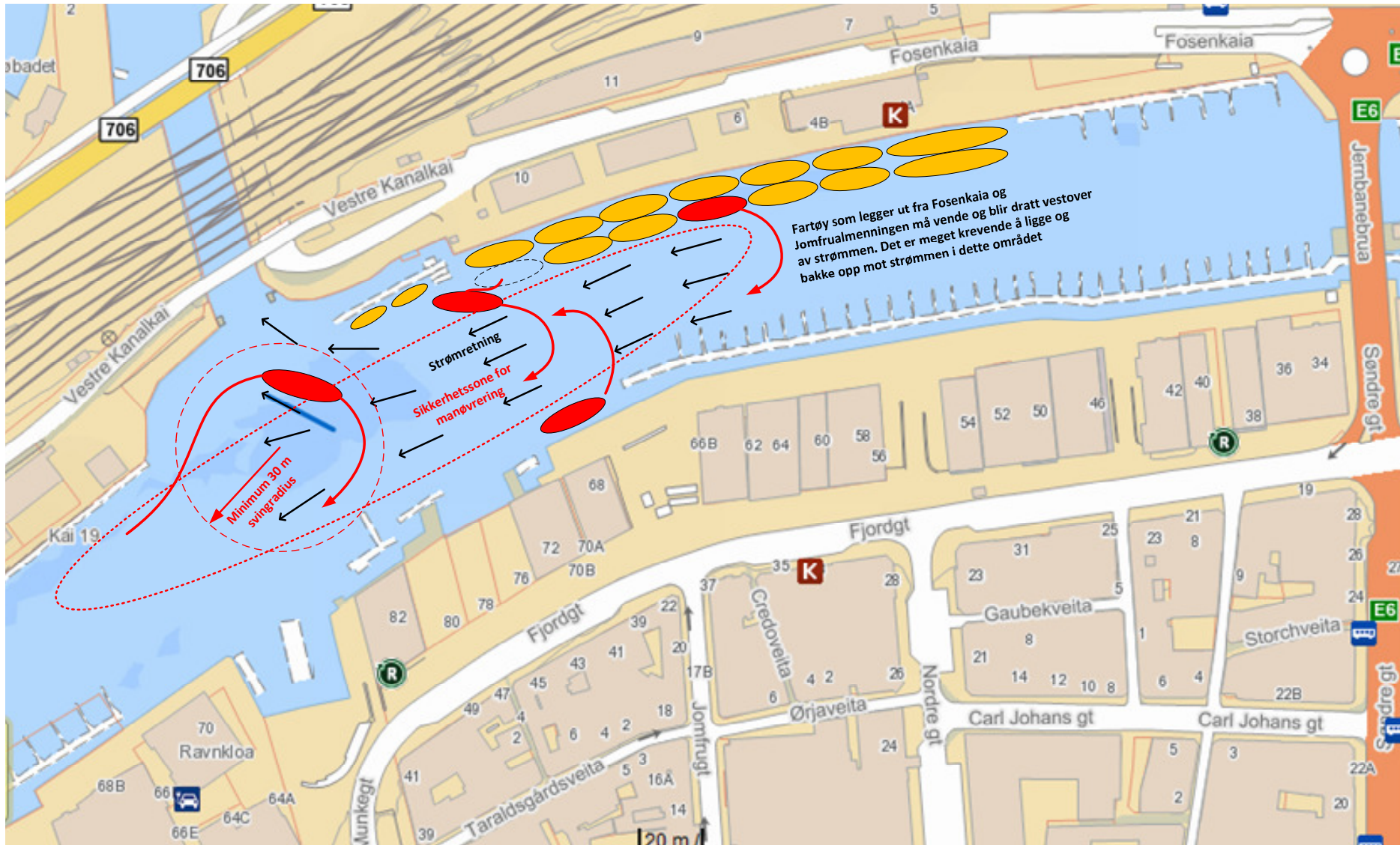
Vedlegg 2. Situasjonsskisse for Kanalen med sikkerhetssoner for manøvrering i farleden.
